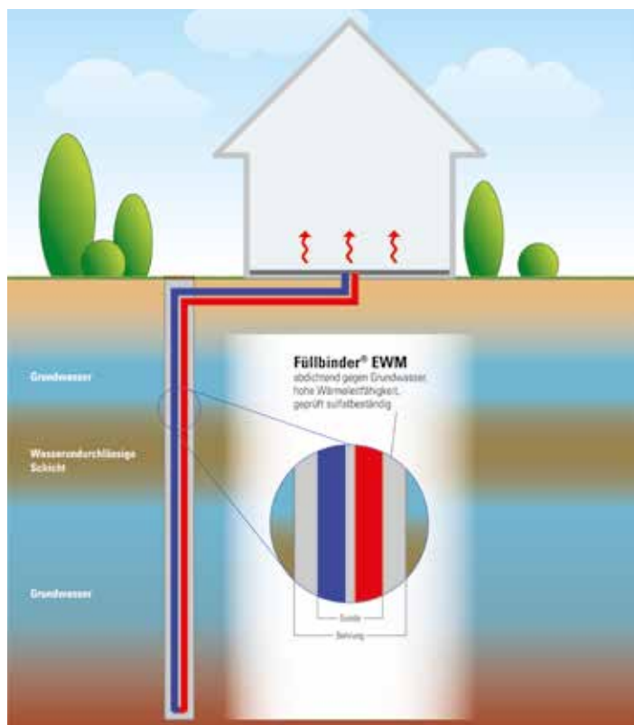
Schematische Darstellung einer Erdwärmesonde
