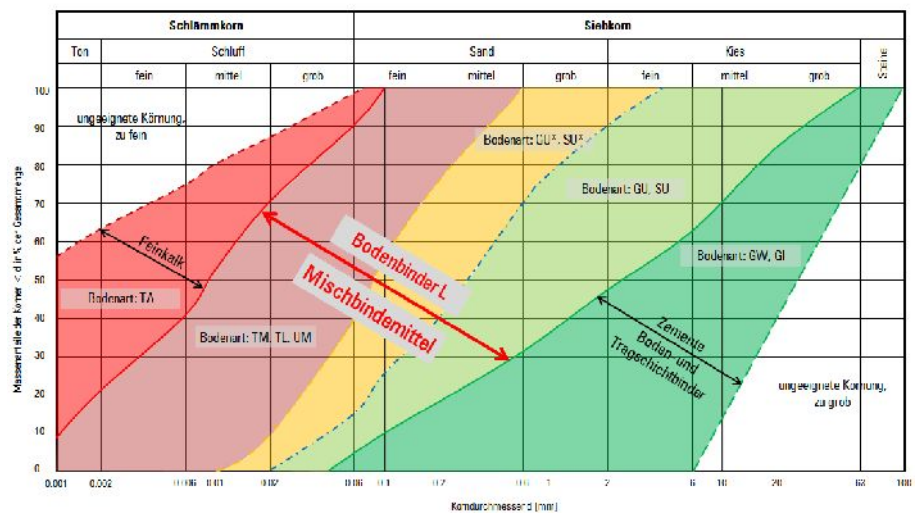
Bindemittelwahl und Anwendungsbereiche anhand der Korngrößenverteilung
